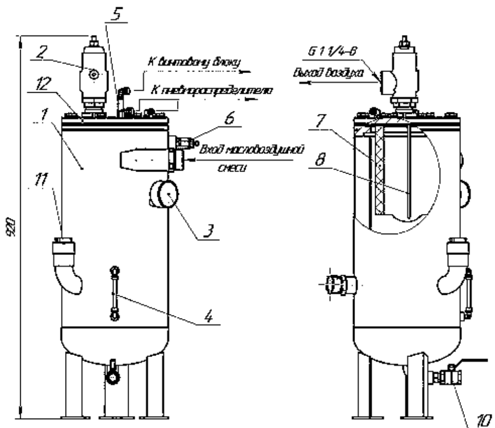
Рисунок 5. Маслоотделитель.
