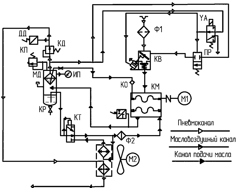
Рисунок 9. Схема пневмогидрокинематическая.
