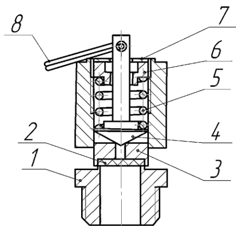
Рисунок 7. Клапан предохранительный.
