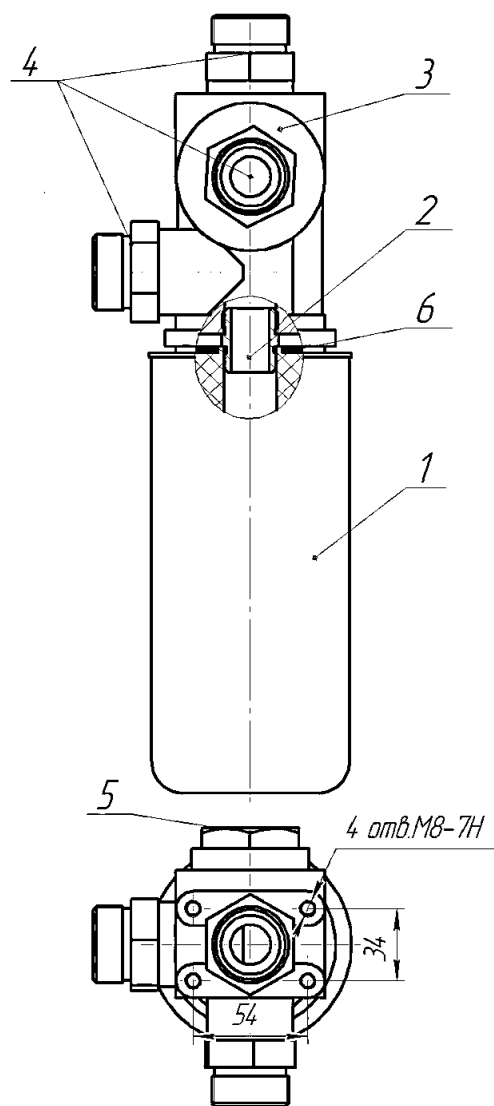
Рисунок 8. Блок распределения.
